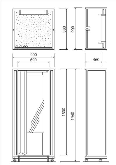
正面図・側面図
