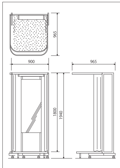
正面図・側面図
