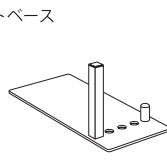
● カットベース (右用) □ SP10-SBR 290×120mm t:5mm (クロームメッキ)
