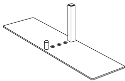
● 基本ベース □ SP10-BS 450×120mm t:5mm (クロームメッキ)
